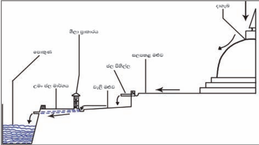
රූපය 1.10 අභයගිරි දාගැබට හා සලපතළ මළුවට වැටෙන ජලය, පොකුණකට ගලා යාමට සලස්වා ඇති ආකාරය
