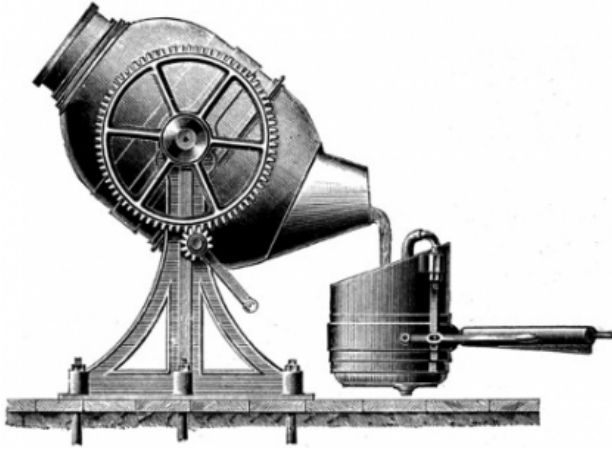
உரு 1.3 ஹென்றி பேஸ்மரின் உருக்கு உற்பத்தி உலை
